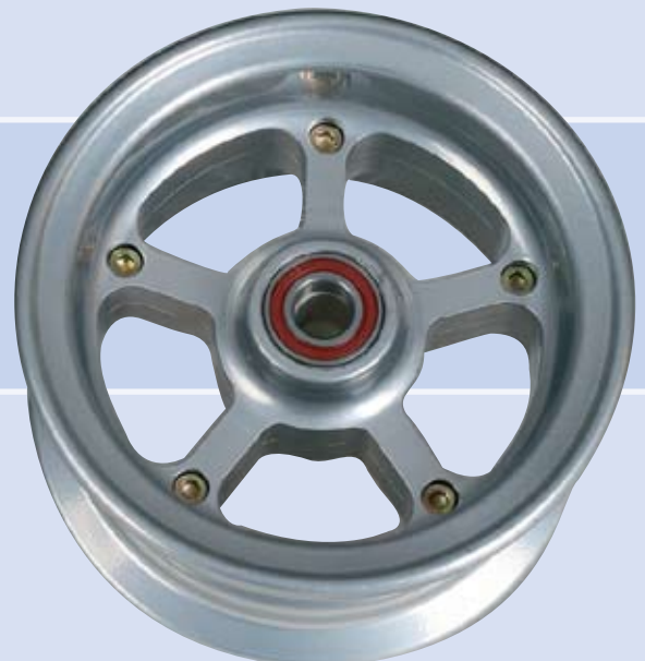
K-106A-000 Nose wheel 6" standard/ Bugrad 6" standard Weight/Gewicht: 1.010 g Price/Preis: 200,80 EUR
